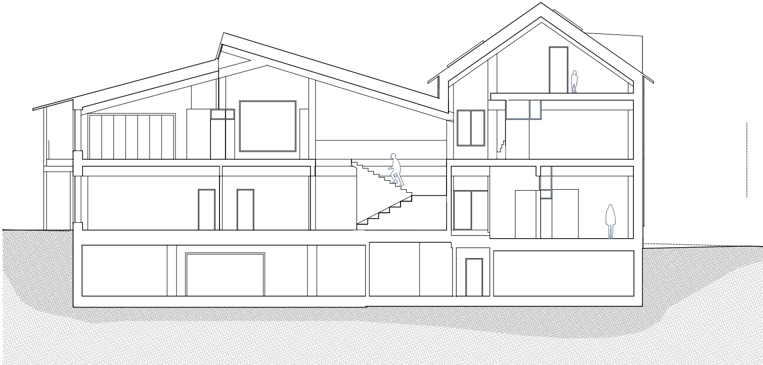
Querschnitt S/1
