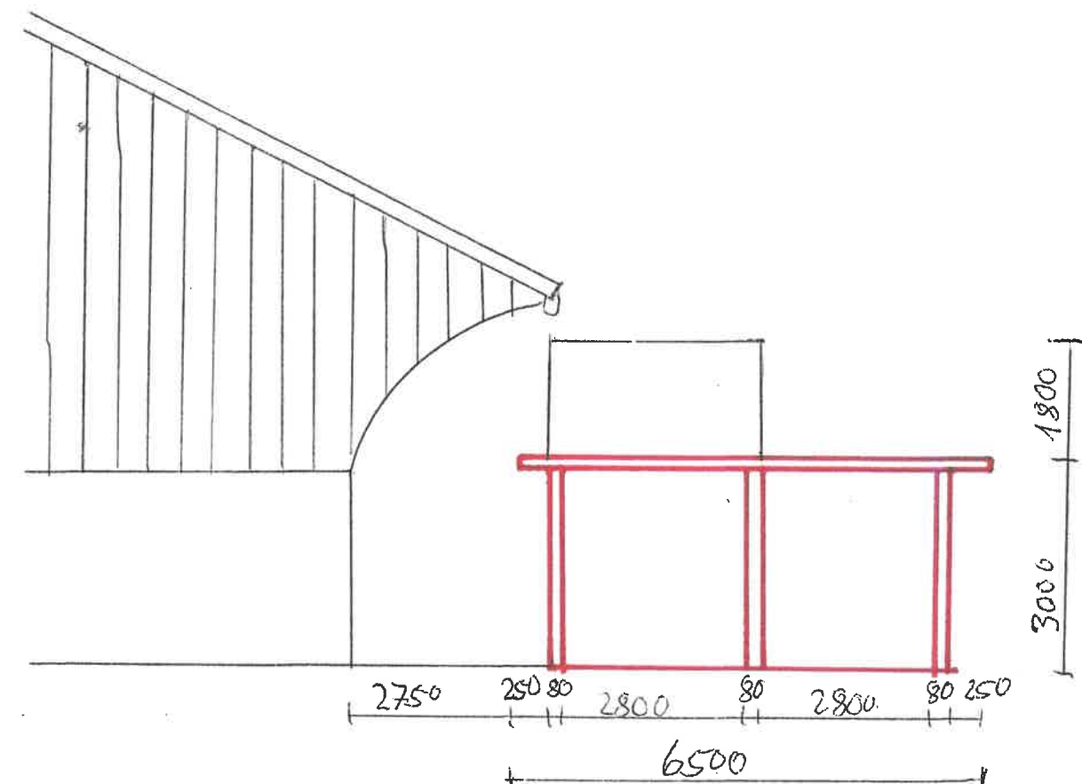
Ansicht Hofplatz
